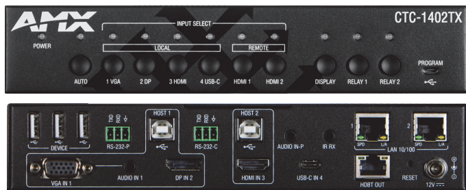
CTC-1402 TX
